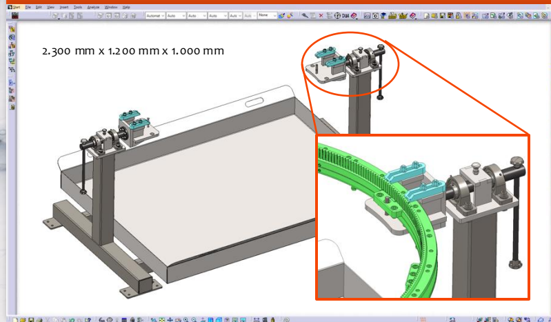
Drehvorrichtung
