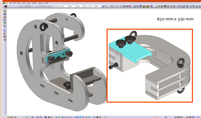
Richthilfsmittel
