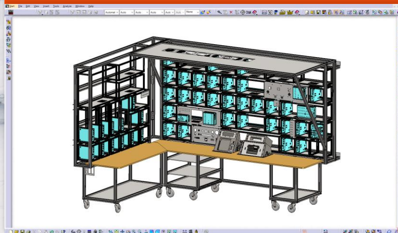
Prüfstand
