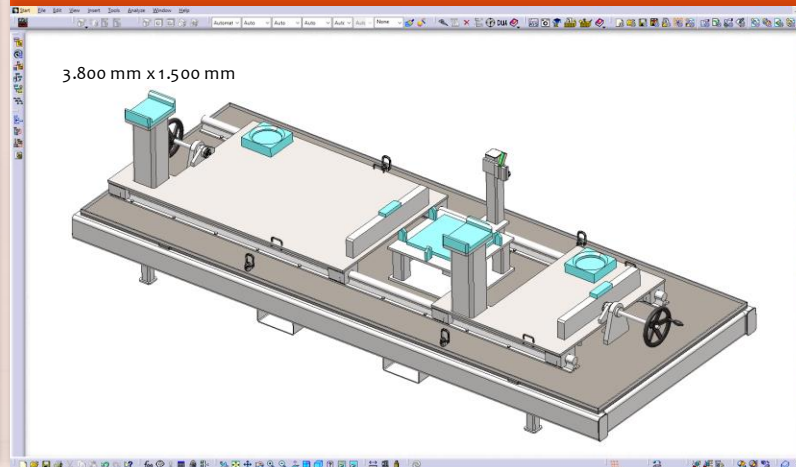
Montagevorrichtung
