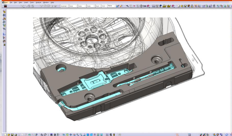
Einleger Bordwerkzeug
