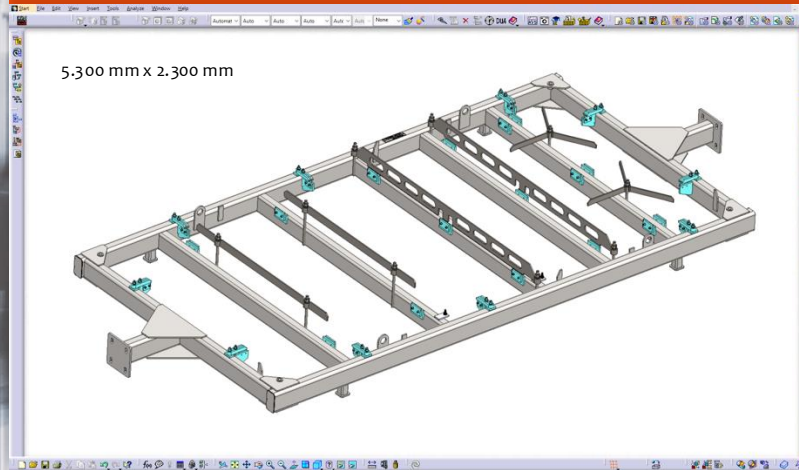
Drehvorrichtung
