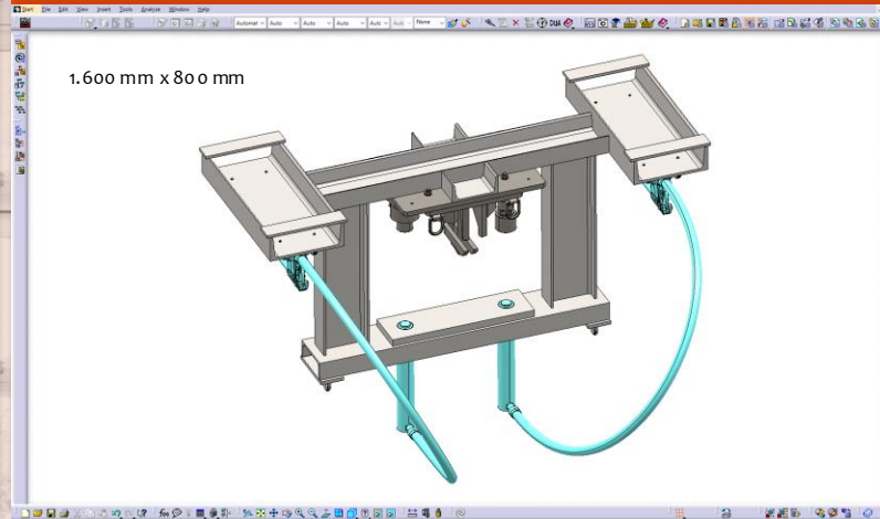
Montagevorrichtung
